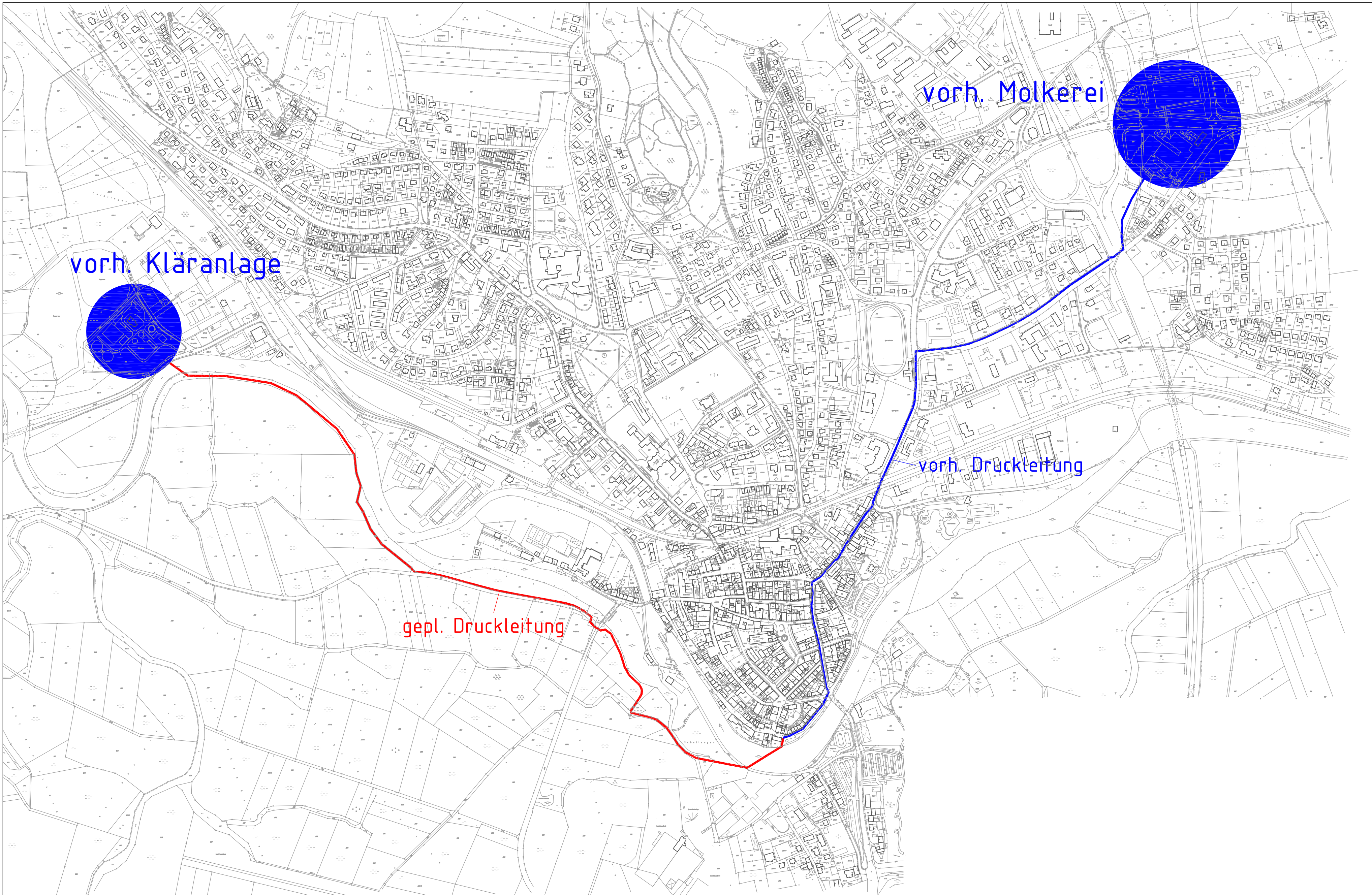
Übersichtslageplan
