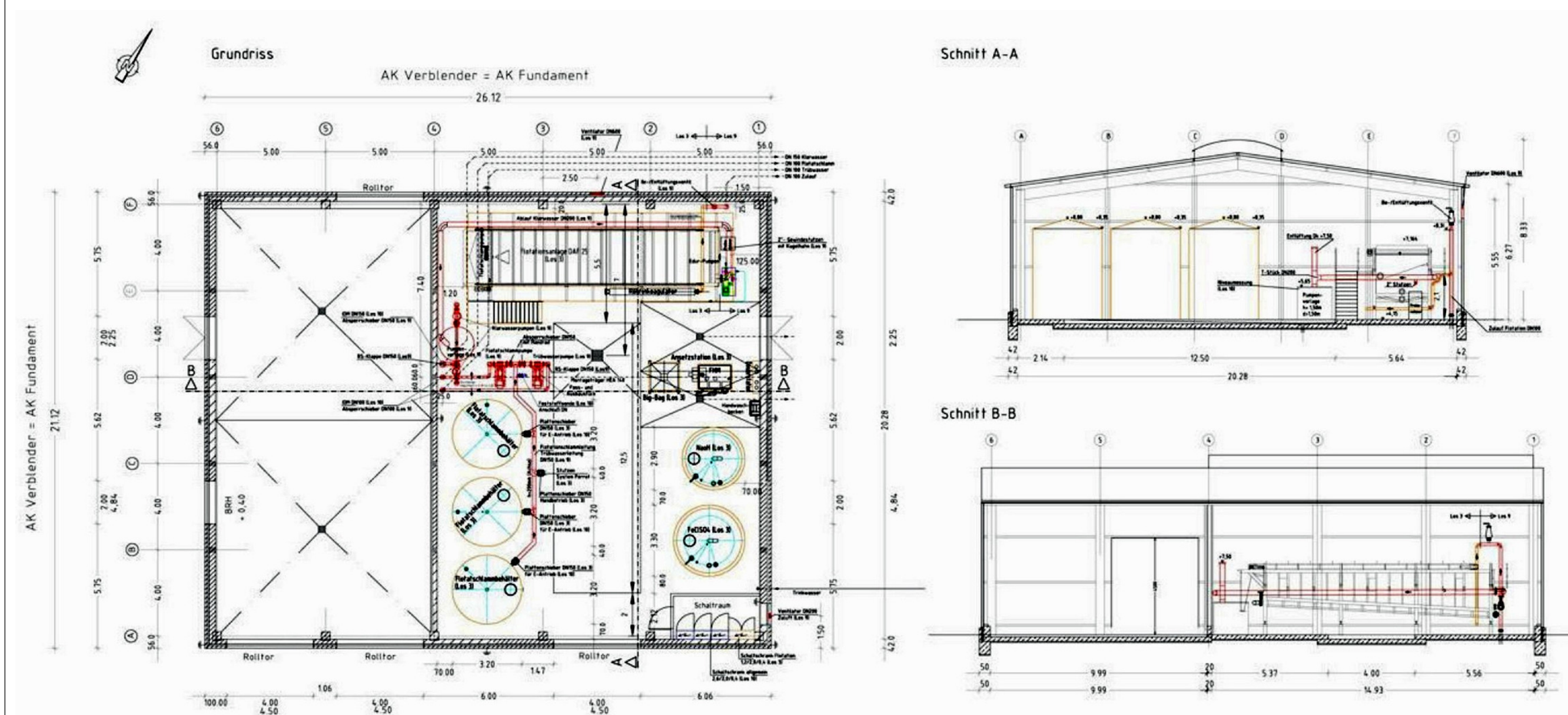
Vorentwurf Flotationsanlage
